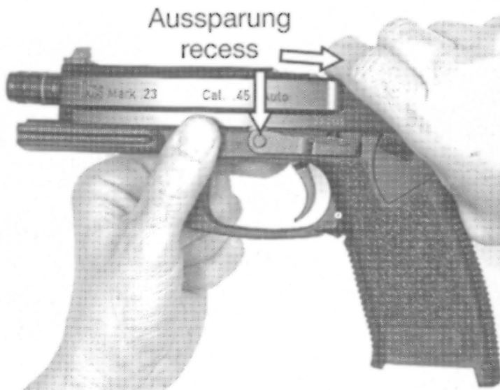
Lage Aussparung zu Verschlussfanghebel Position of the recess of the slide release
