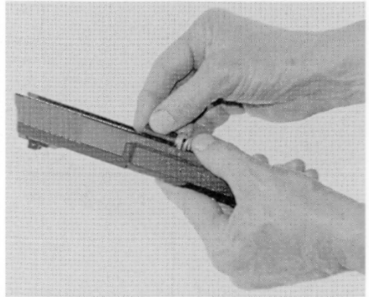
Pufferstange einlegen
